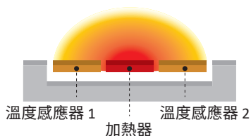
(a) 無流量
