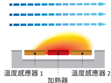
(c) 大流量
