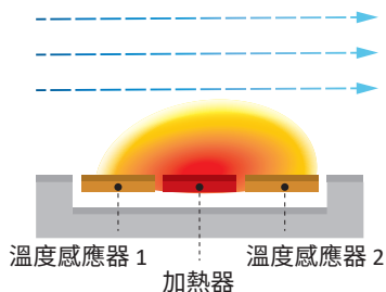
(b) 小流量
