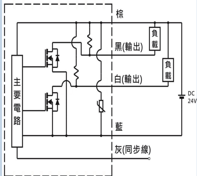
IEY-X45N 接收器(2 組 NPN)
