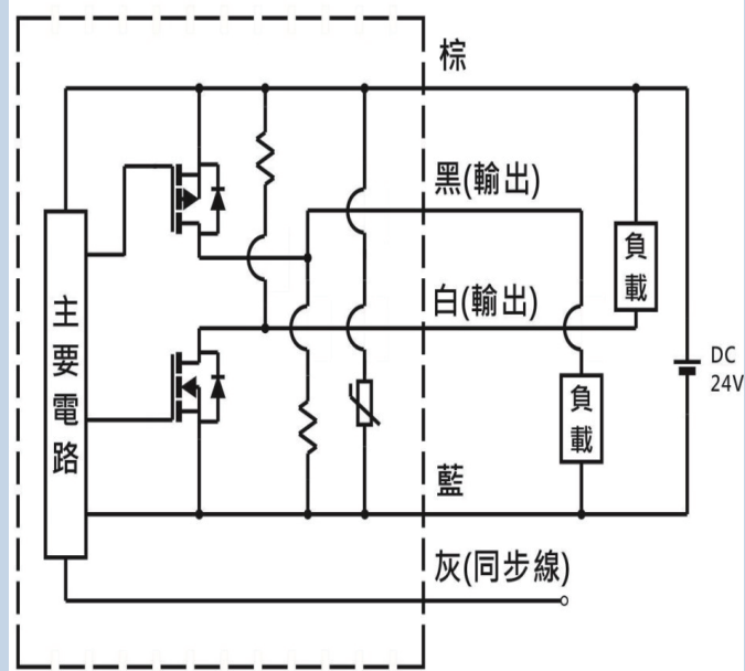
IEY-X45P 接收器(2 組 PNP)
